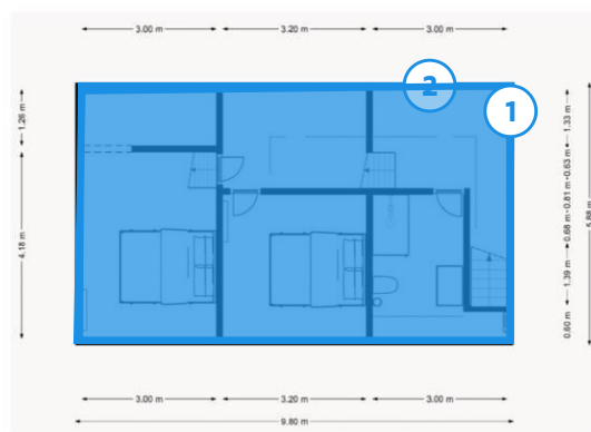
Zième étage
